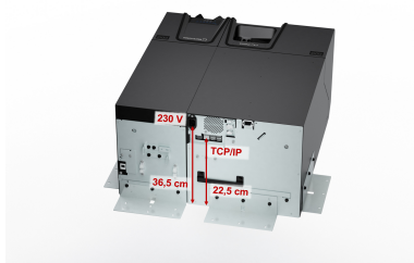
CI-5, Kabelanschluss am Automaten
