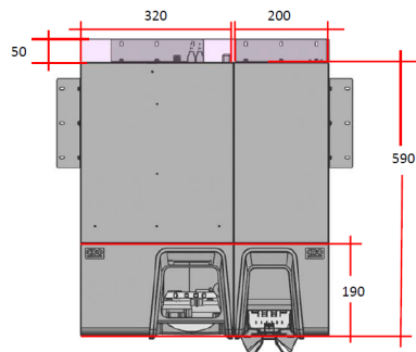
CI-5 technische Zeichnung, Draufsicht
